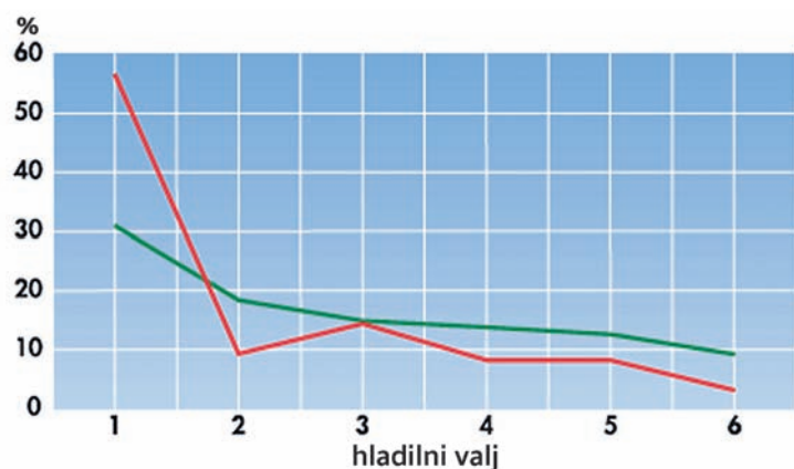
Slika 9. Ohlajanje traku na hladilnih valjih. Grafični prikaz kaže dober (zeleno) in slab profil (rdeče) ohlajanja. Pri konfiguraciji s šestimi valji na prvem ne smemo odvzeti več kot 30 odstotkov toplote.
