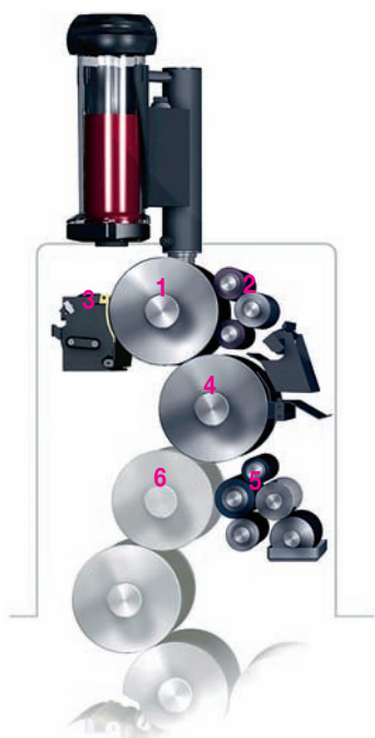
Slika 4. Barvilni sestav Anicolor: 1 - rastrski valj, 2 - sestav treh valjev za doseganje optimalnega ravnovesja tiskarske barva-vlažilna raztopina in čiščenje, 3 - zaprt sestav z rakljem, 4 - barvilni valj, 5 - slojni alkoholni vlažilni sestav Alcolor, 6 - ploščni valj.
