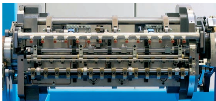
Slika 3. Sistem za obračanje pol med tiskom ima en obračalni bobn dvojnega premera. Zgoraj stranski ris, spodaj fotografija bobna s prijemalci.
