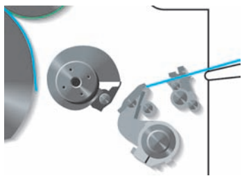
Slika 4. Ekscentrični prenosni valj za manjše upogibanje pol pri predaji z vlažne mize.
