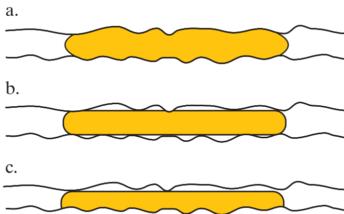
Slika 5. Omočenje lepljenja: a) dobro omočenje – površina obeh lepljencev je v kontaktu z lepilom, b) slabo omočenje – lepilo ima visok kontaktni kot glede na kontaktni kot površine lepljenca, c) povprečno omočenje – samo ena od površin je omočena.
