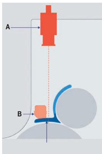
Integrirani kolorimeter Inpress Control meri odtise v stroju namesto na nadzorni mizi. Prihrani najmanj čas za odvzem vzorčnih odtisov.
