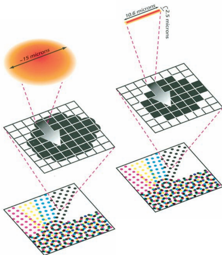
Slika 4. Rastrska pika, zgrajena iz okroglih elementarnih točk.
