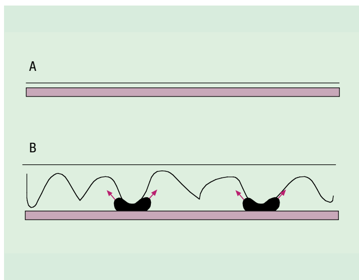
Slika 5. Deformacija nanosa tiskarske barve na gladek tiskovni material (a) in negladek (hrpav) tiskovni material (b) 10 .
